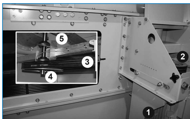
Sistema di azionamento con motore esterno
