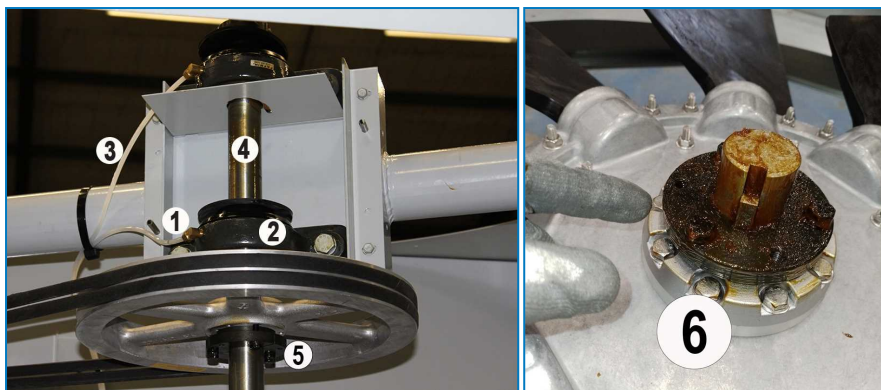
Расположение подшипников вала вентилятора и смазочных фитингов
